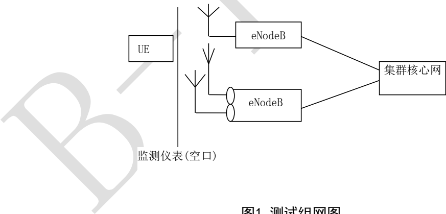
图1 测试组网图
